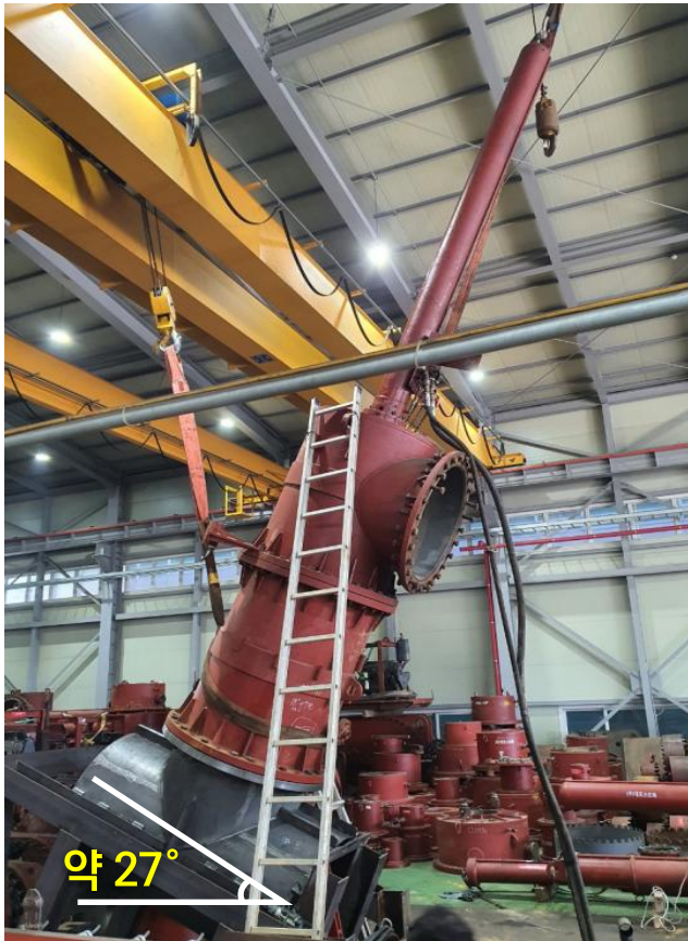
부단수 차단 1500A 성능 테스트
